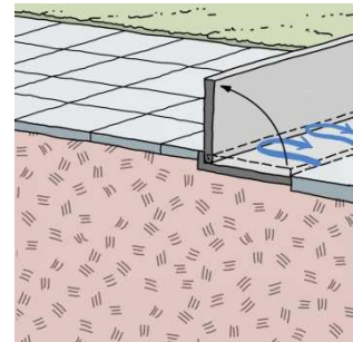
Klappschott
