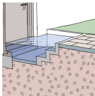
wasserdichte Tür
